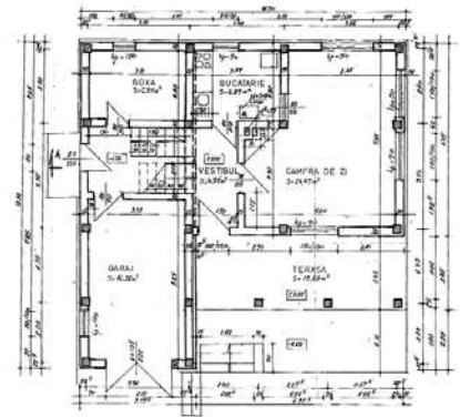
Vilă Voinești, vedere, plan parter
