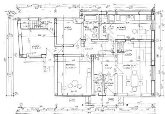
Casă Tânganului, vedere, plan parter
