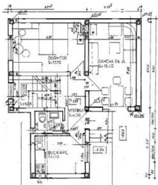
Vilă Plaurului, vedere, plan parter
