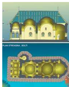
Biserica Mogoșoaia, secțiune, plan streaișină, vedere
