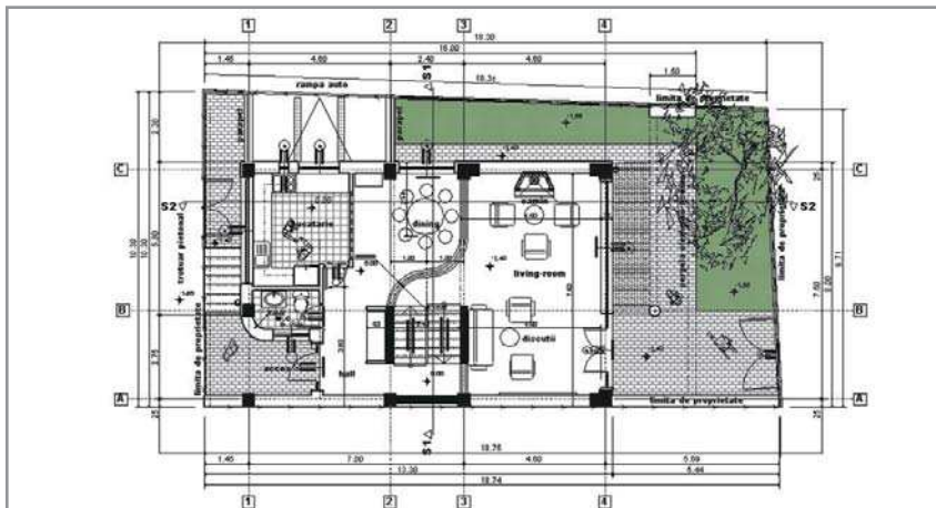
Casa Cornescu - plan parter
