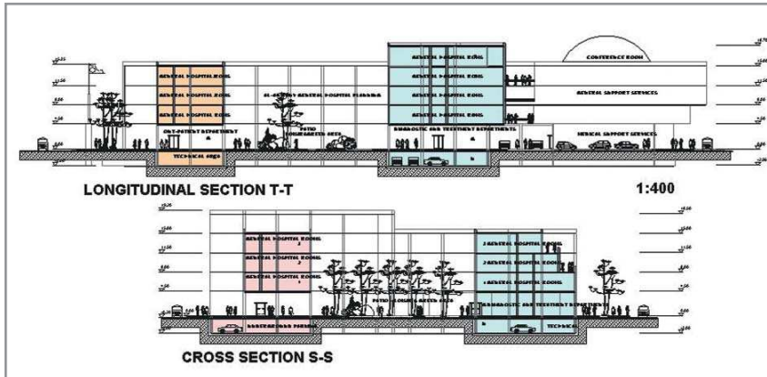
Spital în Arabia Saudită
