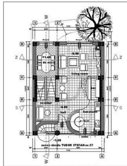
Casă str. Tudor Ștefan - plan parter
