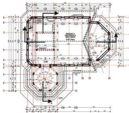
Biserică ortodoxă vedere, plan
