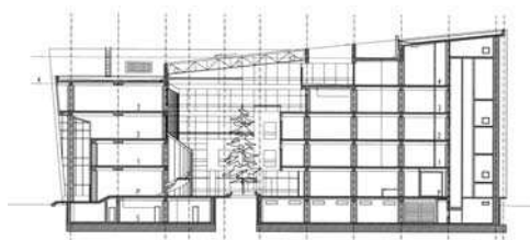
Primăria sector 2 București vedere, secțiune, plan parter
