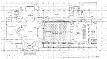
Casa de cultură Snagov, vedere, plan parter
