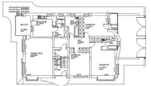
Locuință București, perspectivă, plan parter
