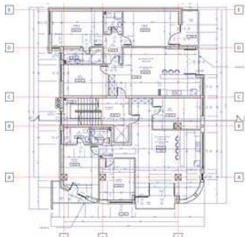
Imobil str. Glinka, perspectivă, plan etaj 1
