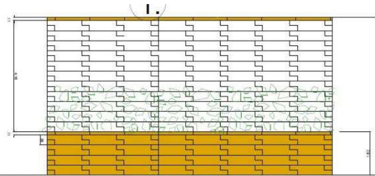
Sectione AA
