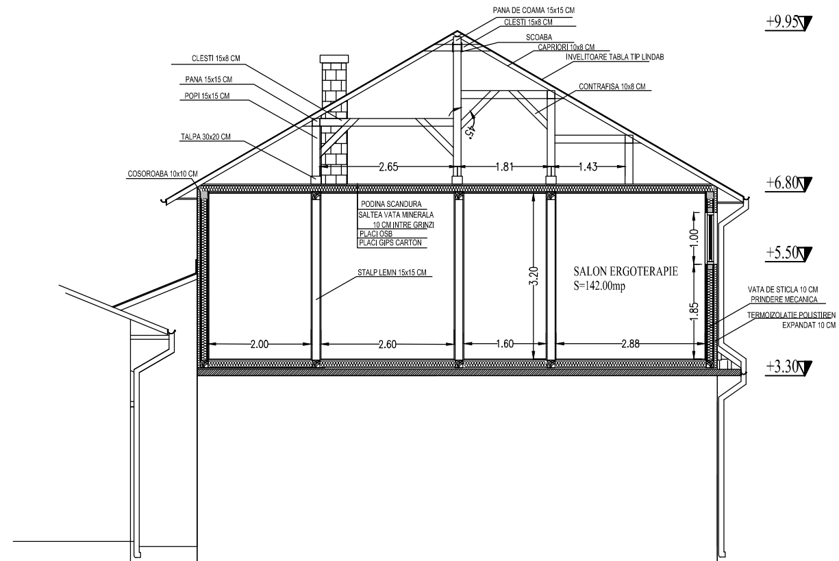
SECTIUNE TRANSVERSALA SC. 1/100
