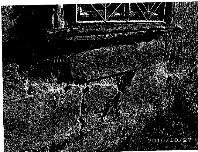
Foto 47 – Degradarea tencuielilor și zugrăvelilor la fațadă (parapetul ferestrei)
