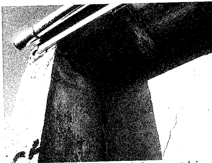
Foto 37 – Fisurarea și desprinderea peretelui calcan al corpului lateral dreapta
