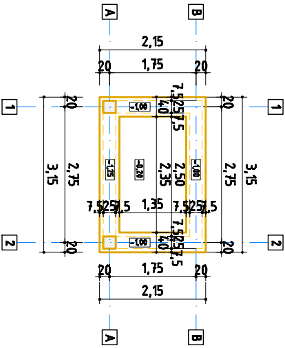
PLAN FUNDATII
