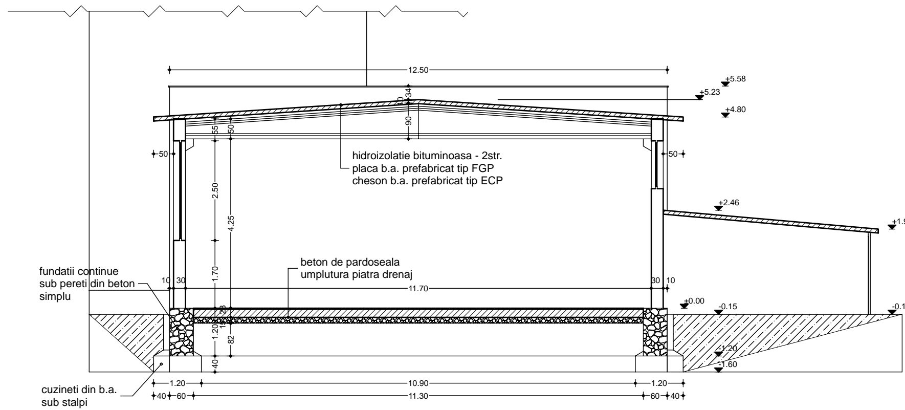
SECTIUNEA 1-1
