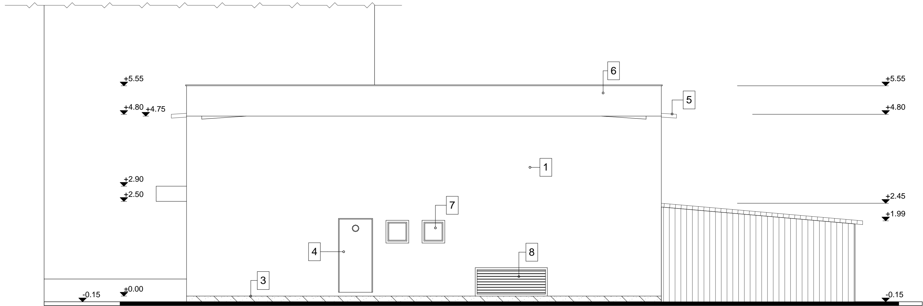
FATADA EST
