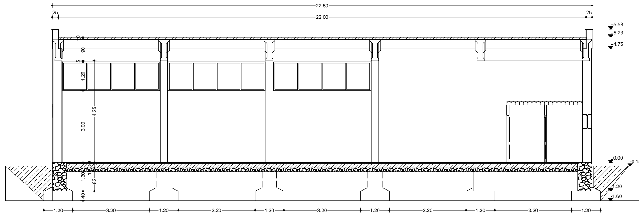
SECTIUNEA 2-2
