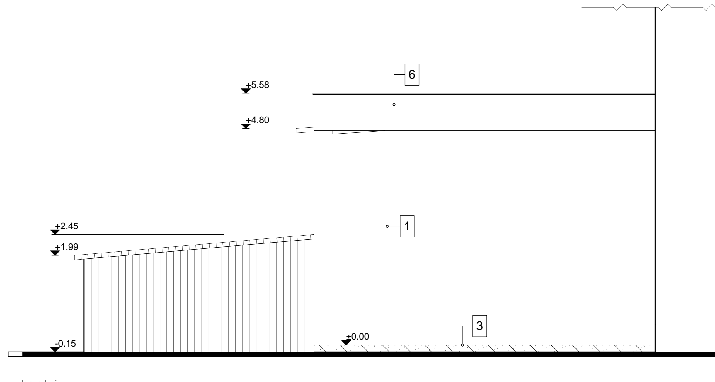
FATADA NORD
