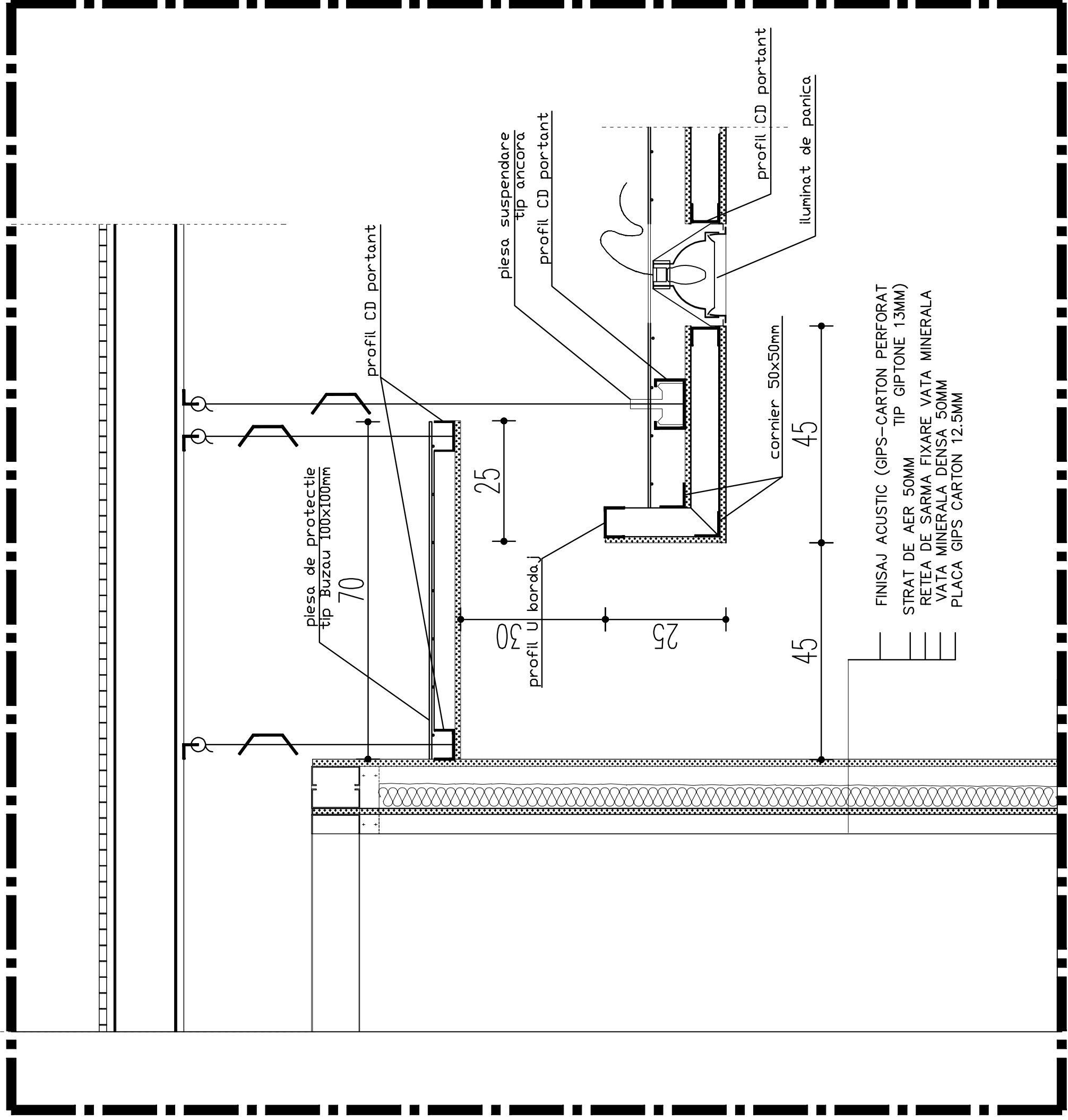
DETALIU SCAFA FUM SALA SPECTACOLE
