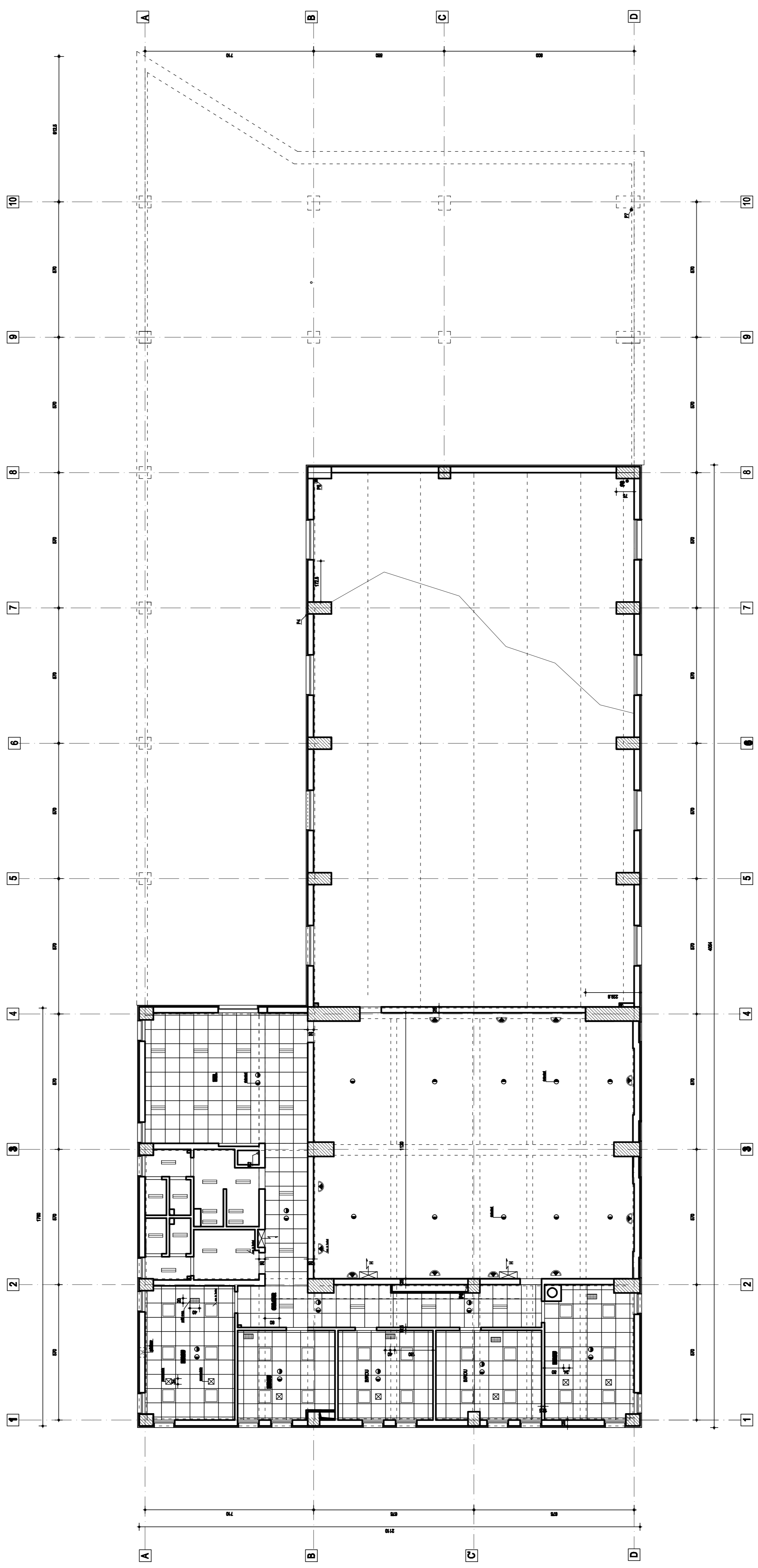
PLAN PLAFONETAJ 2
