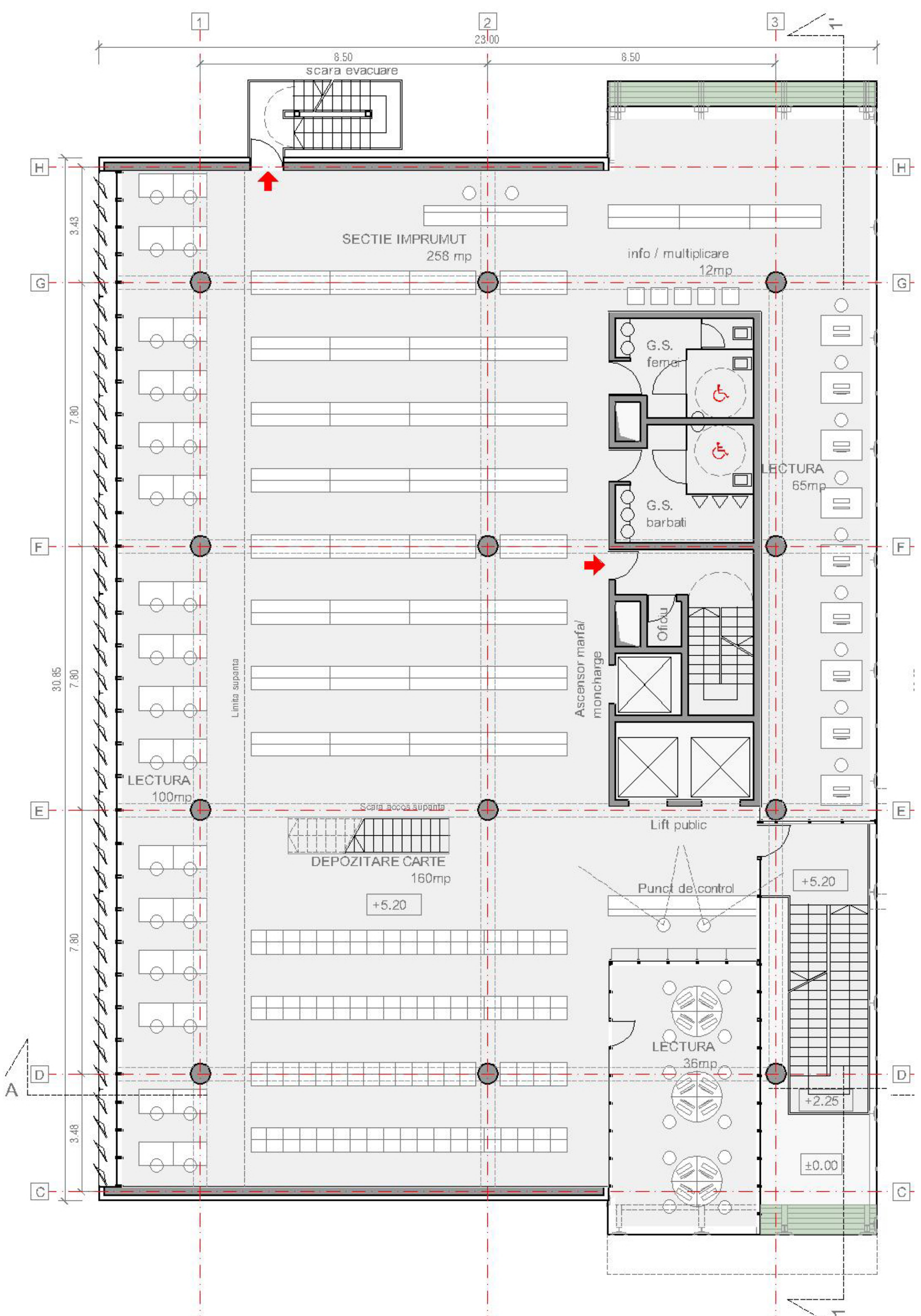
PLAN ETAJ 1 SC. 1:100
