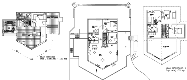
Casă Provița de Jos, vedere, planuri
