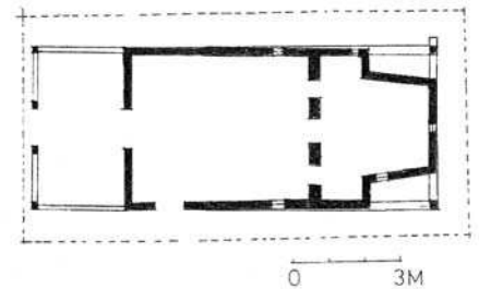
Mănăstirea "Bunavestire" Valea Cormăii, Bistrița-Năsăud - strămutare, consolidare, restaurare vedere, plan
