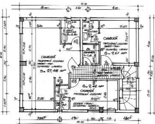
Spațiu comercial vedere, plan etaj 2
