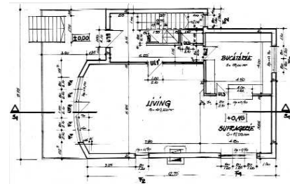
Vilă unifamilială vedere, plan parter
