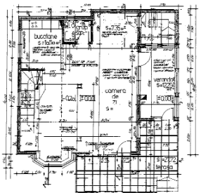
Locuință unifamilială vedere, plan parter
