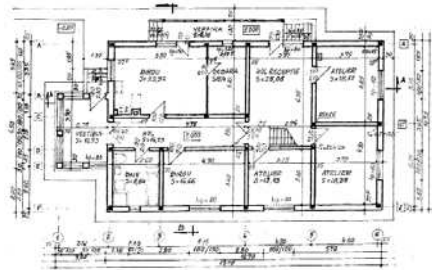
Vilă Brașov, vedere, plan parter
