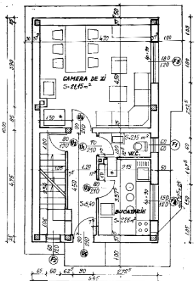
Vilă Bușteni, vederi, plan parter
