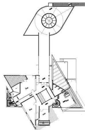
Locuință - colecție de artă „Ștefan Râmnicăneanu” aleea Teișani, București, măchetă, plan parter
