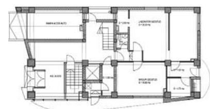
Imobil apartamente și spații comerciale str. Polonă nr. 56 - București, vedere, plan parter
