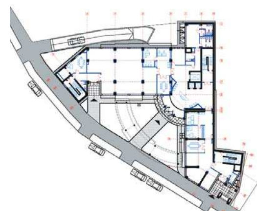
Clinica franco-română str. Sf. Vineri, vedere, plan parter
