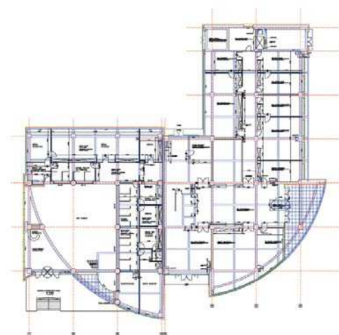
Sediul Romgaz, vedere, plan parter
