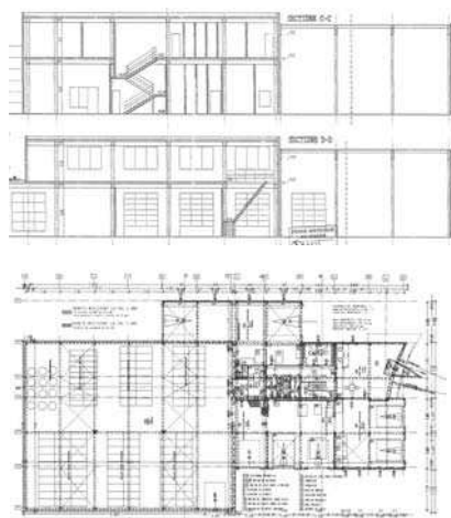
Centru Comercial Marsorom, secțiuni, plan
