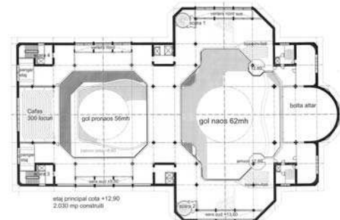
Concurs 2002 – Catedrala Mântuirii, machetă, plan etaj
