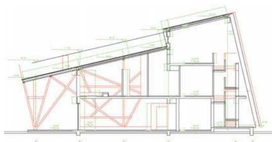
Locuință str. Jandarmeriei, vederi exterior, interior, secțiune
